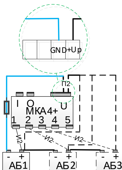
Рис.9. Схема подключения МКА4+ с кабелем П2 с 1,2 или 3-мя АБ 12В либо с 2- или 3-мя АБ 6В. Вместо комплектных кабелей И2 с июля 2026г. поставляются их модификации И2В .
