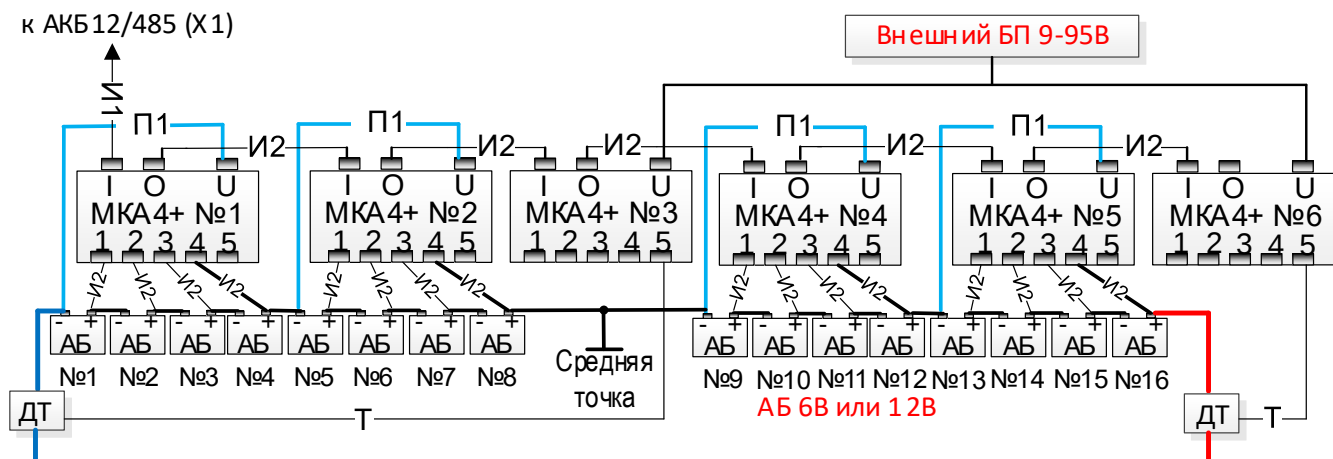
Рис.7. Пример схемы для мониторинга цепи аккумуляторов 6В или 12В со средней точкой. Вместо комплектных кабелей И1, И2 с июля 2026г. поставляются их модификации И1В, И2В соответственно.
