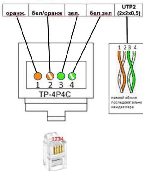
Кабель И1В (МКА4+ ---- АКБ485_12)
