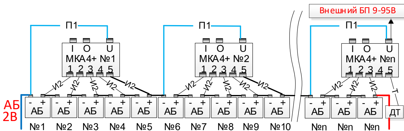
Рис.10. Пример мониторинга цепи АБ 2В обязательно по 5 шт. на 1 МКА4+ при питании их от АБ. Вместо комплектных кабелей И1, И2 с июля 2026г. поставляются их модификации И1В, И2В соответственно.
