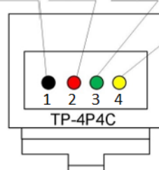
Кабель И2 (МКА4+ --- МКА4+; МКА4+ --- КТРJ)
