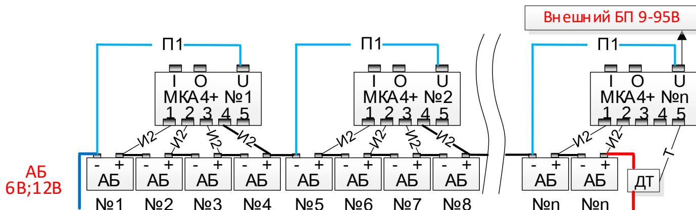
Рис.8. Пример подключения АБ 6В или 12В по 4 шт. на 1 МКА4+. Вместо комплектных кабелей И2 с июля 2026г. поставляются их модификации И2В .
