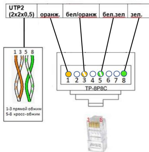
Кабель И1В (МКА4+ ---- АКБ485_12)
