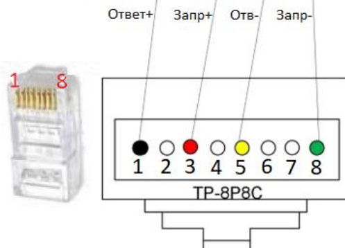
Кабель И1 (МКА4+ ---- АКБ485_12)
